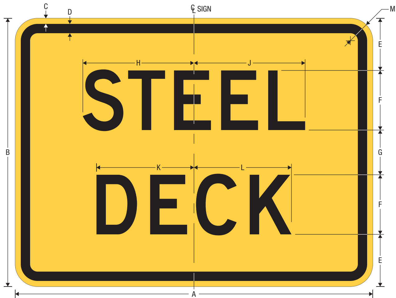
W8-5bP STEEL DECK (PLAQUE)
